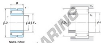
NA49, NA59
